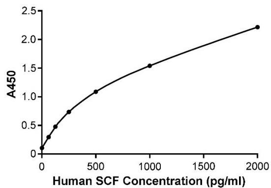
图3. Human SCF ELISA Kit的标准曲线。实测数据会因实验条件、检测仪器等的不同而存在差异，图中数据仅供参考。
